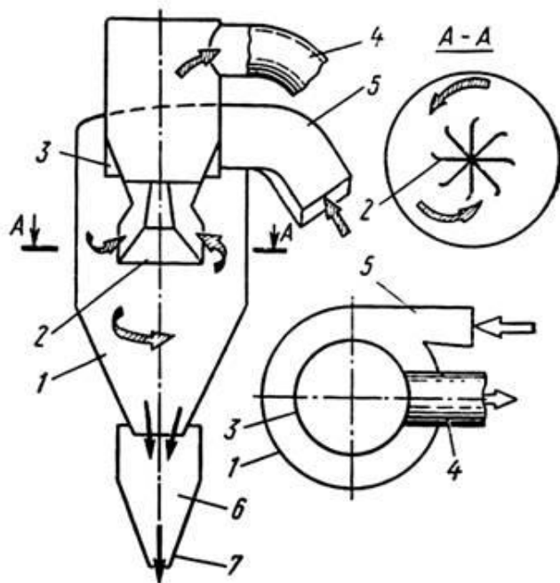
Рисунок 47 – Схема устройства пылевого циклона
