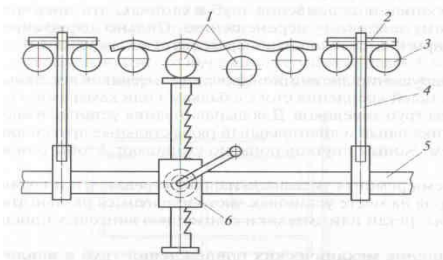
Рисунок 13 – Рихтовка труб экрана реечным домкратом
