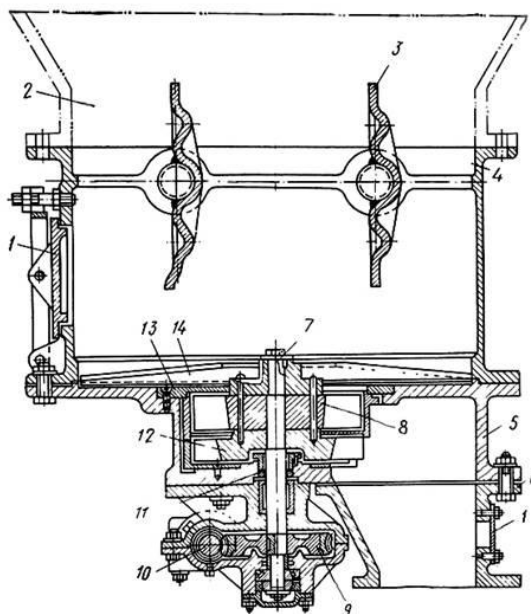
Рисунок 44 – Лопастной питатель пыли
