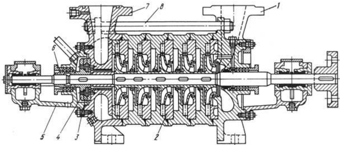
нок 49 – Насос секционного типа
