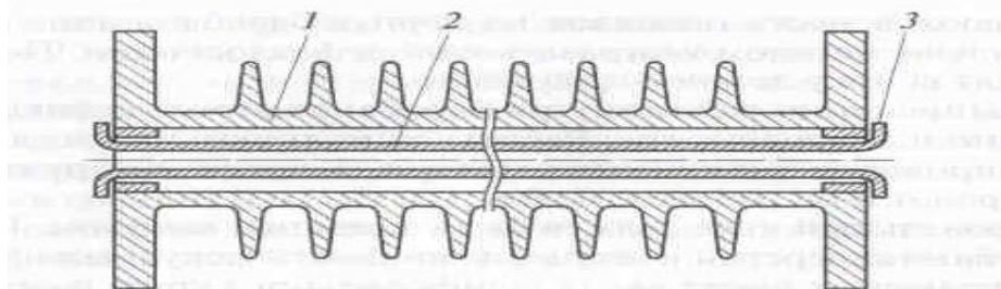
Рисунок 20 – Ремонт ребристой трубы вставкой стальной трубы
