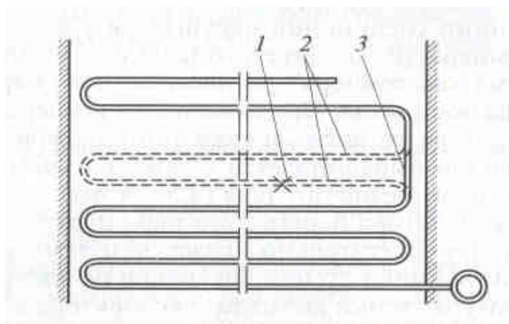
Рисунок 14 – Установка закоротков на змеевике
