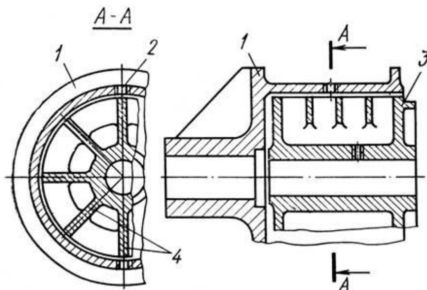
Рисунок 27 – Дробевая муфта
