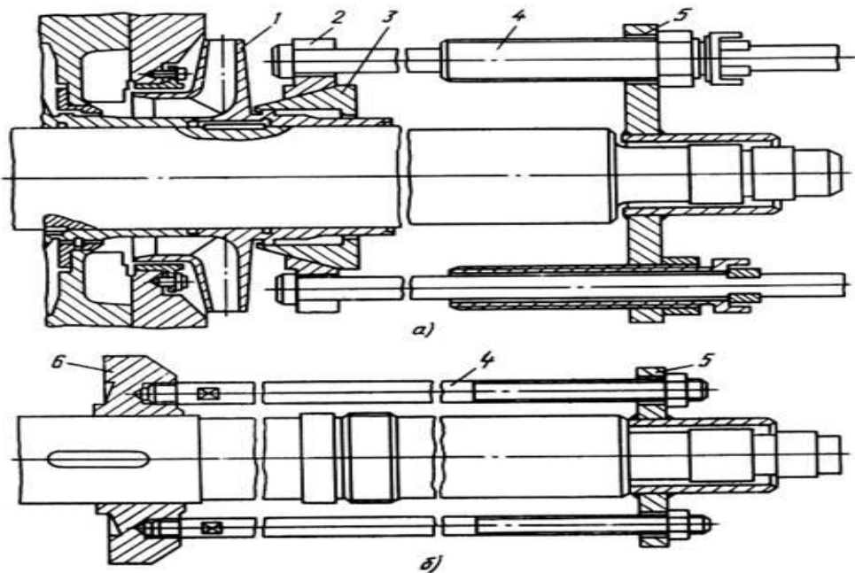
Рисунок 50 – Приспособления для снятий деталей с вала насоса
