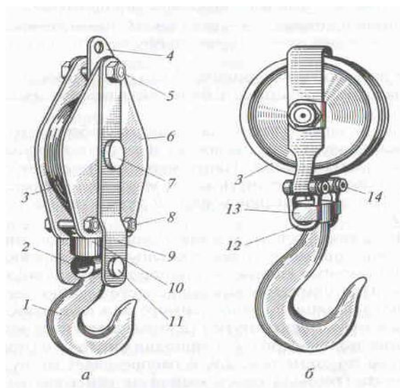
Рисунок 7 – Блоки для стальных канатов
