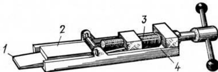
Рисунок 37 – Клиновой домкрат для центрирования валов
