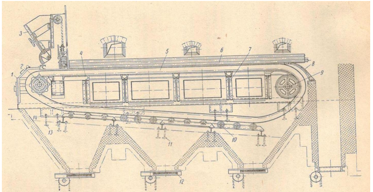
Рисунок 22 – Общий вид цепной решетки БЦР-М
