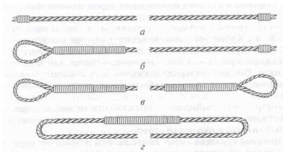
Рисунок 10 – Типы стропов
