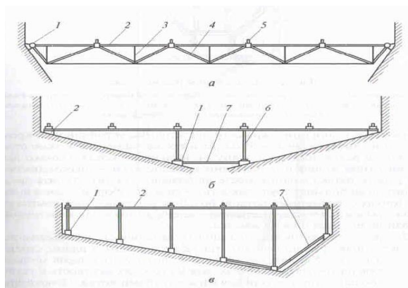
Рисунок 2 – Опорные балки
