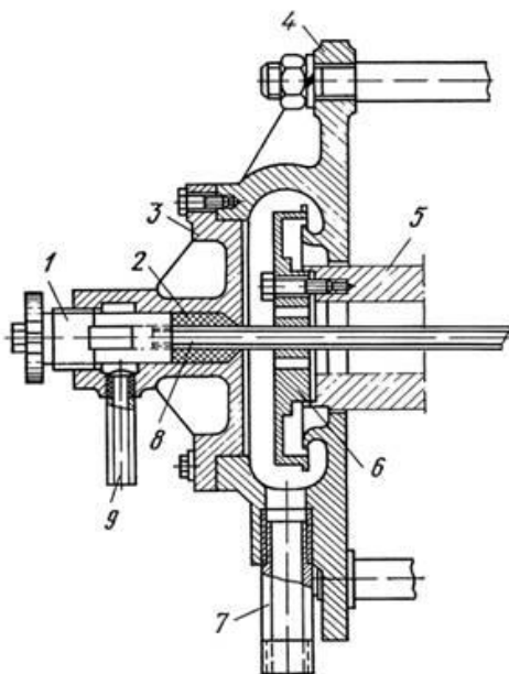
Рисунок 42 – Водораспределительная головка
