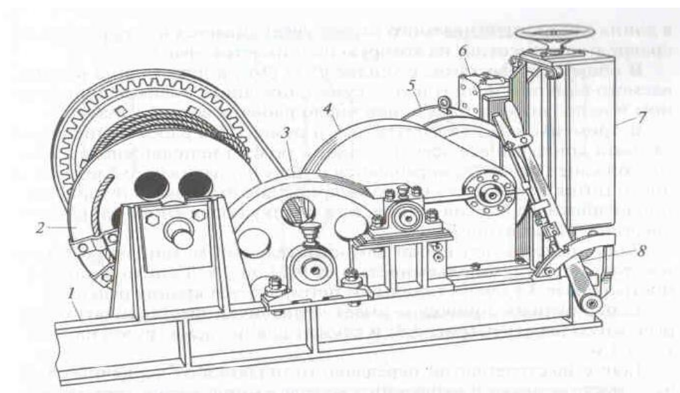
Рисунок 6 – Лебедка с электрическим приводом
